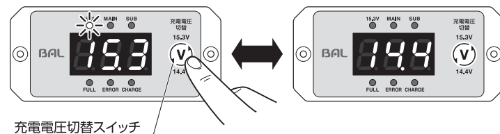
充電電圧切替スイッチ
